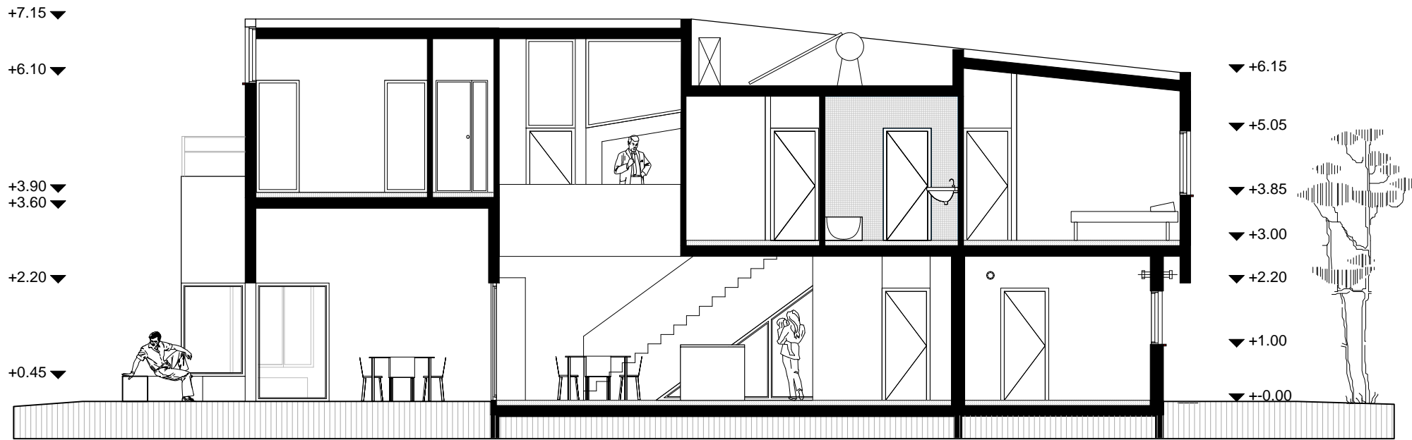
A-A section
