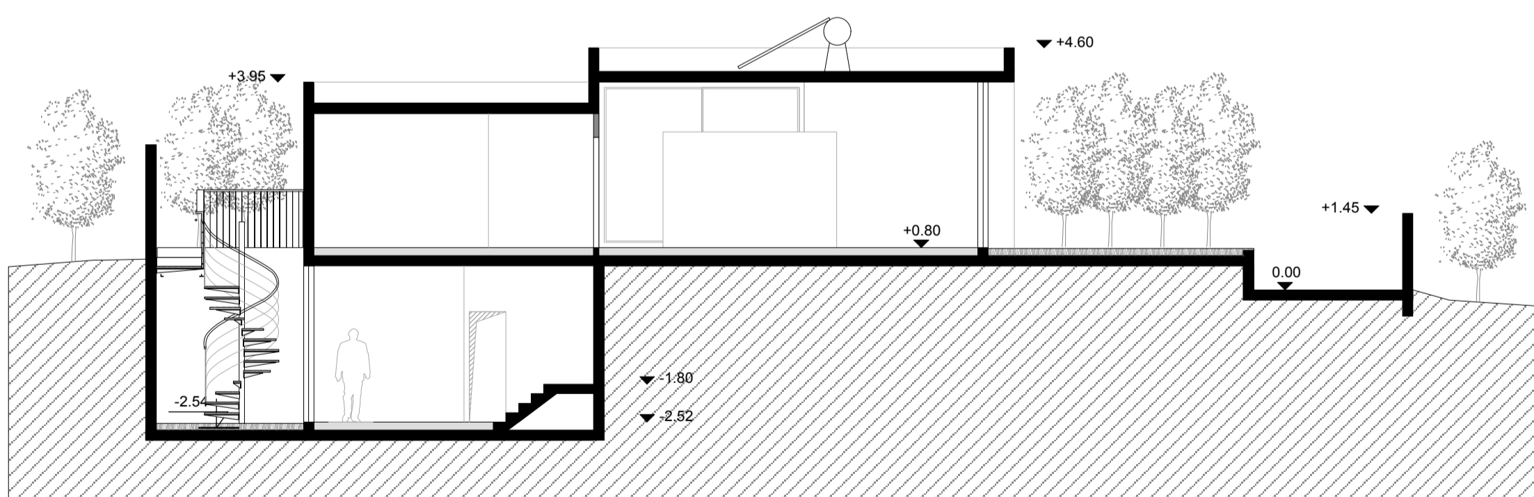
Section D-D
