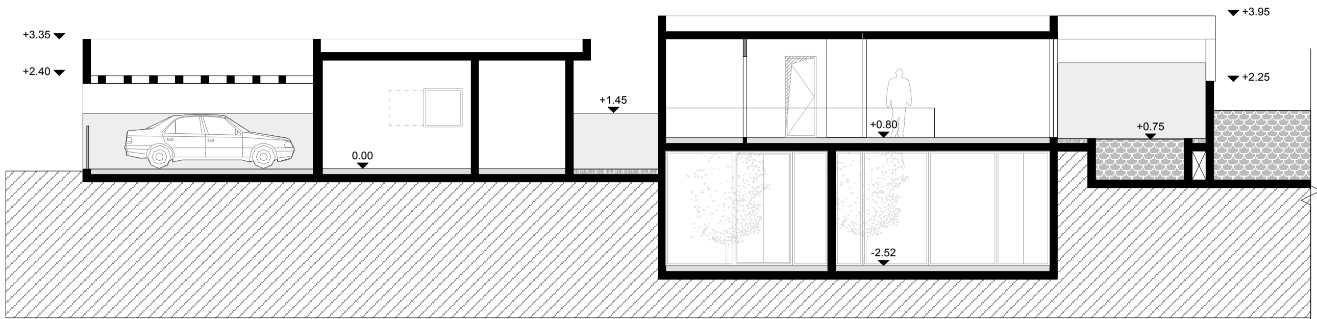
Section A-A
