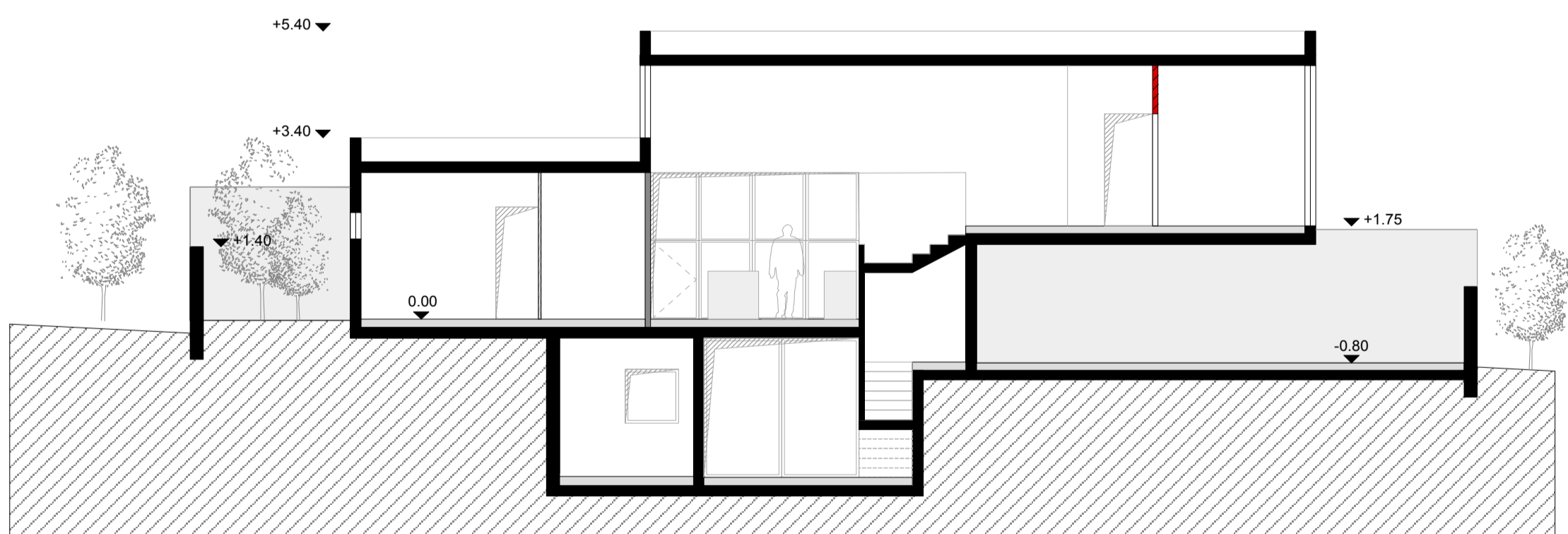
Section D-D
