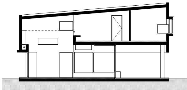
section DD
