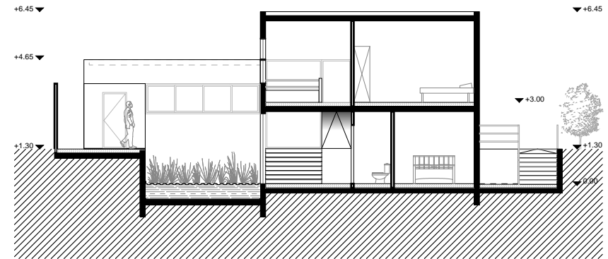
Section D-D
