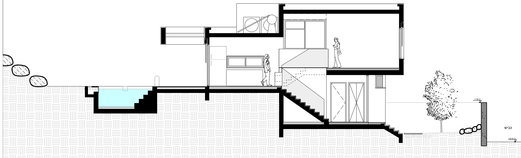
חתך B-B 1:100
