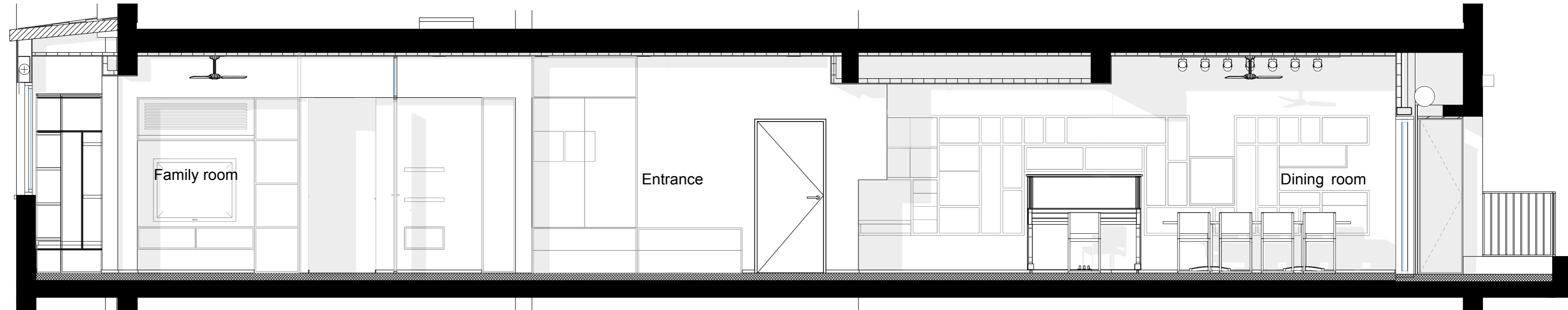
Section A-A
